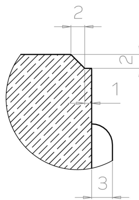
DETALJ B
